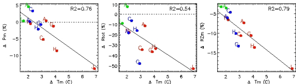
Figure 28 : Relations entre les variations moyennes de température sous CC et les variations associées de précipitations, d'écoulement total et d'humidité de la zone racinaire par rapport au climat actuel. Les lettres réfèrent aux MCG utilisés pour les simulations de CC (A : ARPEGE, C : CCCma, G : GFDL, H : HadCM3, J : CCSR/NIES, L : LMD6, N : NCAR PCM et les points rouges, bleus et verts correspondent aux scénarios d'émission A2, B2 et +1% CO 2 /an.
