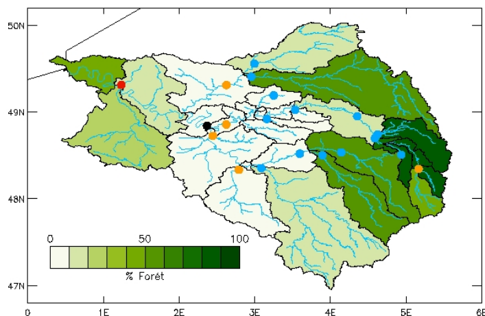
Figure 4 : Discrétisation du bassin versant de la Seine selon CaB, en 29 sous-bassins unitaires. La couleur verte indique le pourcentage de forêt dans notre application. Le réseau hydrographique principal apparaît en bleu, et les points localisent les 20 stations de jaugeage exploitées pour la calibration du modèle (Poses en rouge, Paris en noir).
