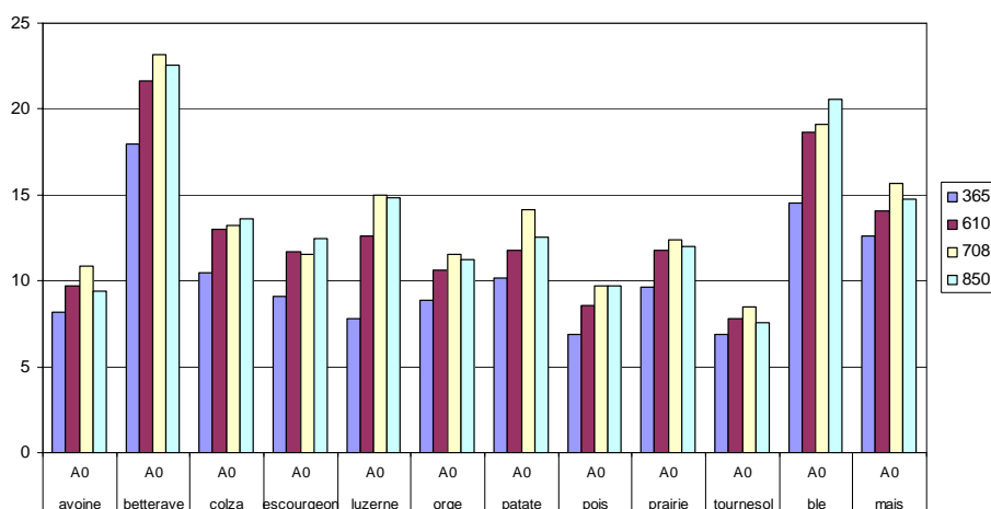
Figure 15 : Production totale de biomasse aérienne par culture (t MS ha -1 ) sous les différents climats considérés : Actuel (365ppm), ARPEGE NEW B2 (610 ppm) et A2 (850 ppm), ARPEGE OLD (708 ppm).
