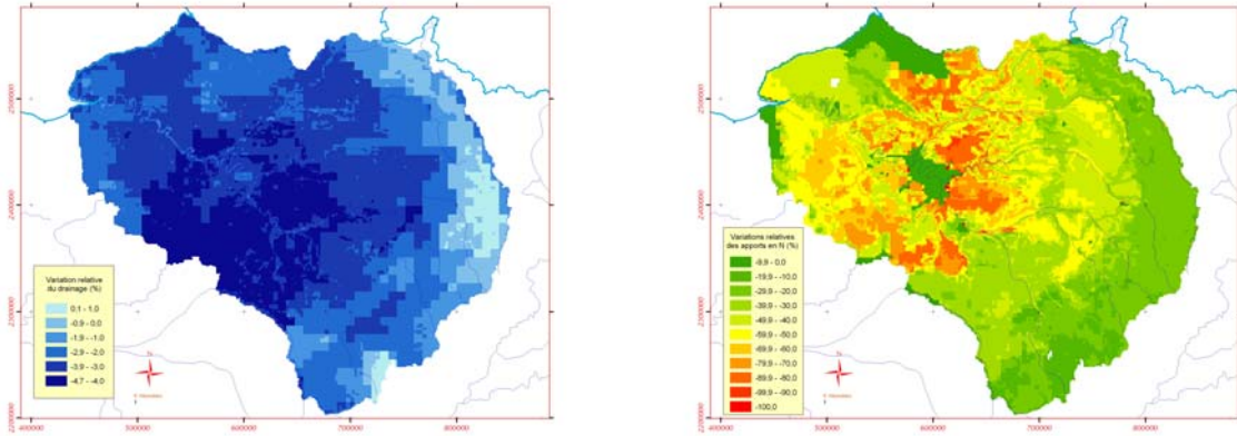
Figure 19 : Variation relative des flux d'eau drainés vers les nappes et des flux de nitrates : rapport agriculture raisonnée / agriculture actuelle, sous climat actuel (moyenne sur 1970-1989).
