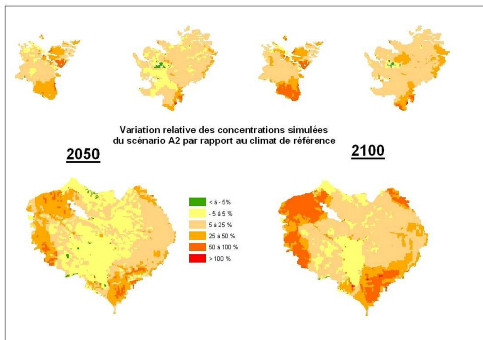
Figure 17 : Variations relatives des concentrations simulées sous scénario ARPEGE NEW A2 par rapport au climat de référence après 50 et 100 ans de simulation.
