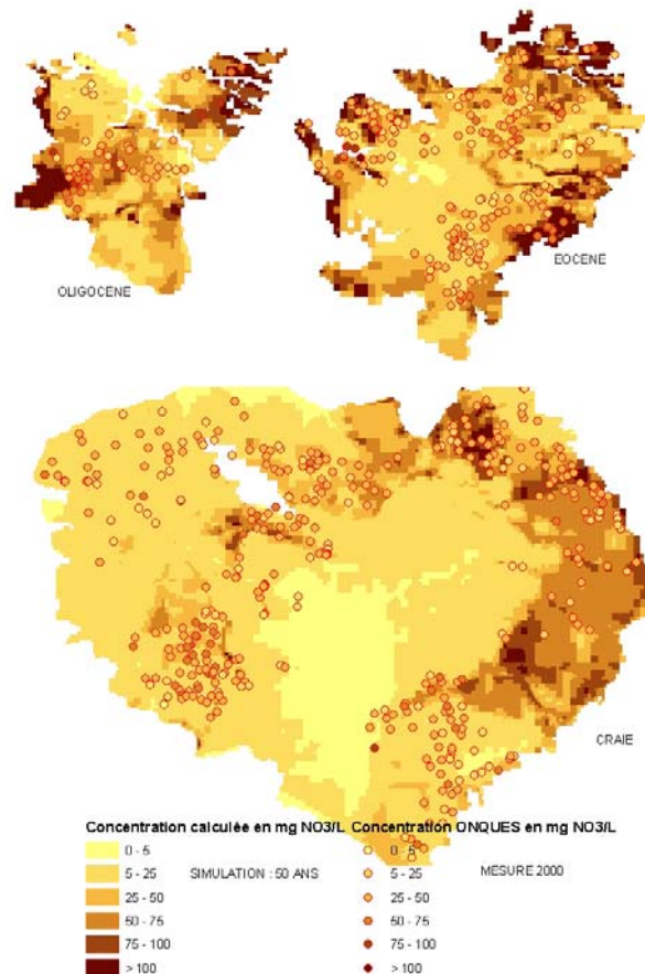
Figure 7 : Concentrations en nitrate calculées (50 années de simulation) et mesurées en 2000.
